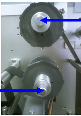
(A)リボン巻取り摘み・リボンブレーキ摘み 時計回り-強 反時計回り-弱
